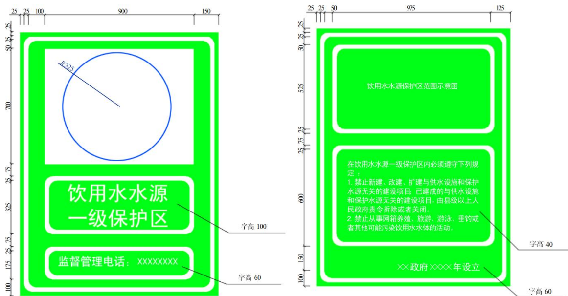
饮用水水源保护区界标正面图示及尺寸 (单位: mm)
